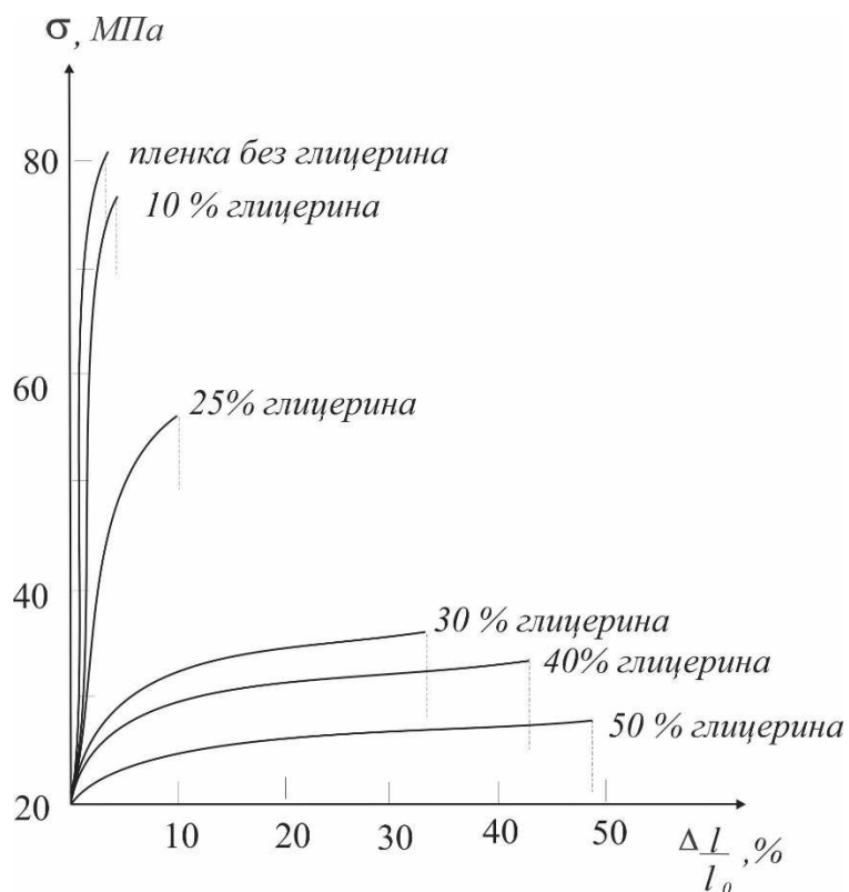
Рис. 1. Зависимость напряжение-деформация для пленок ХТЗ.
